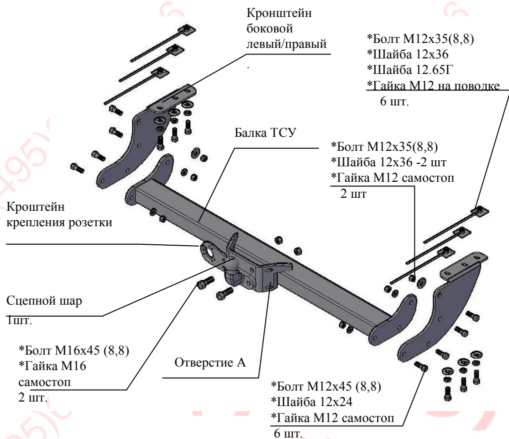
Рис.1 Тягово-цепное устройство 6050 .
